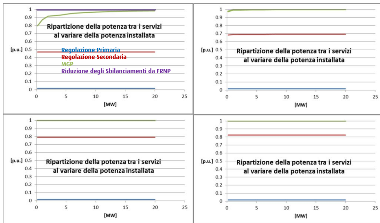
Figura 2.5 – Confronto della ripartizione della potenza nominale del SdA fra i differenti servizi al variare della potenza nominale stessa per le diverse durate considerate – Caso di accoppiamento con PV e installazione in zona NORD
