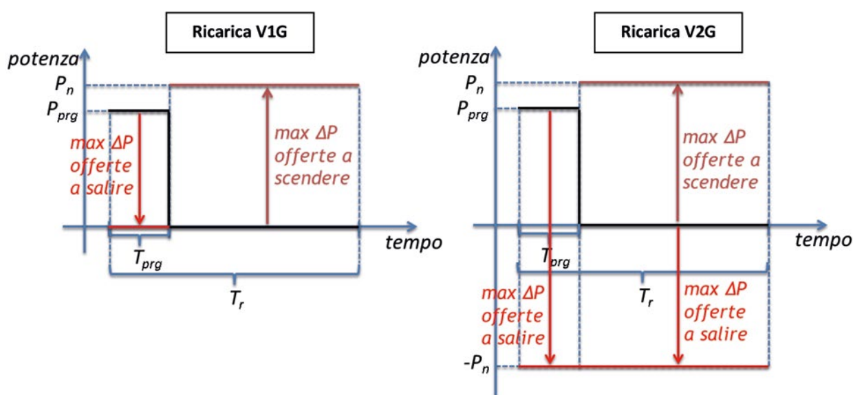
Figura 5.1 - Massima ampiezza in potenza delle offerte simulate per il SB in ciascun periodo di ricarica
