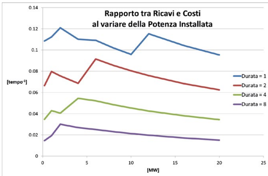
Figura 2.10 – Comparazione dell'andamento del rapporto tra ricavi netti e investimento al variare della potenza installata in funzione della durata del SdA – Accoppiamento con FRNP eolica e installazione in zona CNOR
