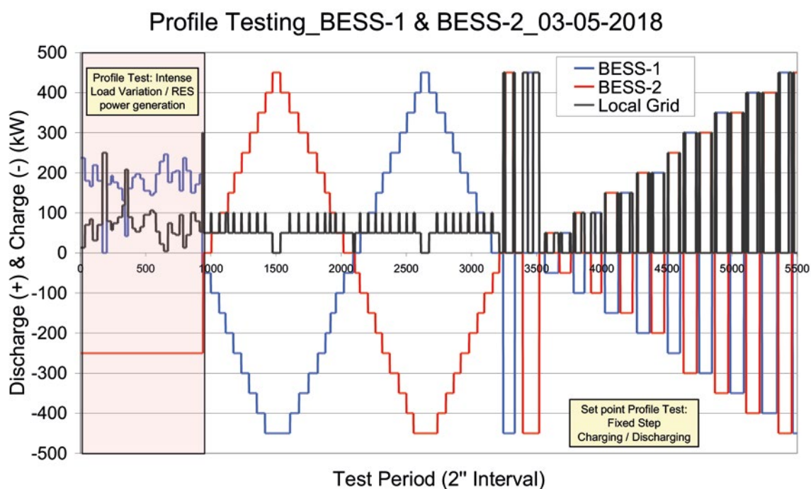
Figura 7.3 - Test del SdA con diversi profili di potenza
