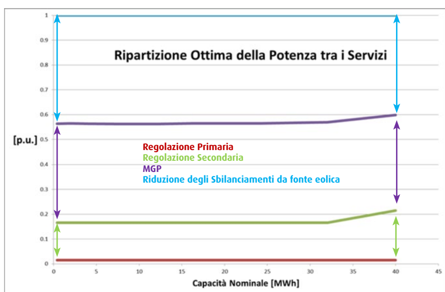
Figura 2.9 – Ripartizione ottima della potenza installata fra i vari servizi al variare della taglia – zona CNOR con accoppiamento ad un impianto eolico
