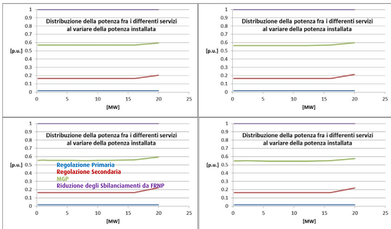
Figura 2.11 – Confronto della ripartizione della potenza nominale del SdA fra i differenti servizi al variare della potenza nominale stessa per le diverse durate considerate – Caso di accoppiamento con eolico e installazione in zona CNOR
