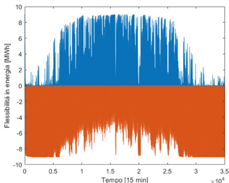
Figura 4.8 - Flessibilità in energia teorica dell'aggregato su un orizzonte temporale di un anno nel caso di sola funzionalità di autoconsumo
