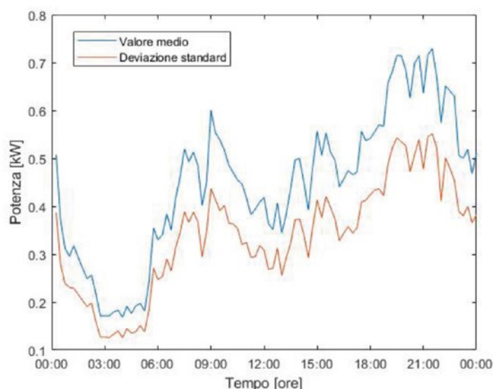
Figura 4.1 - Valore medio e deviazione standard del consumo della popolazione simulata durante ogni quarto d'ora di una giornata feriale estiva
