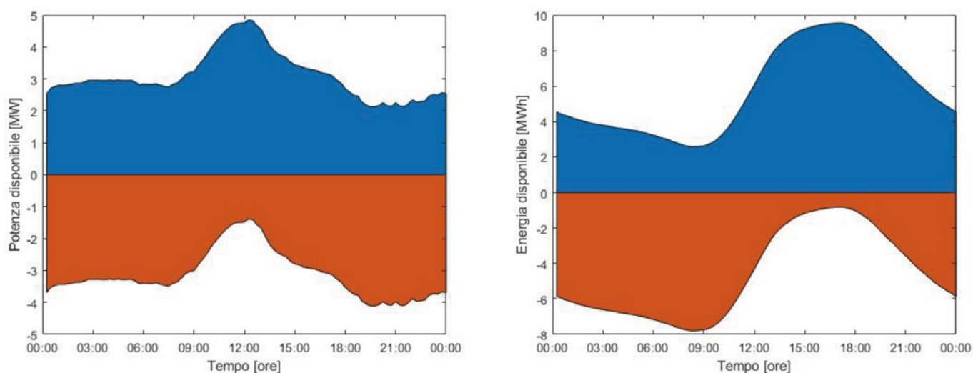
Figura 4.7 - Flessibilità teorica dell'aggregato di una giornata soleggiata feriale estiva
