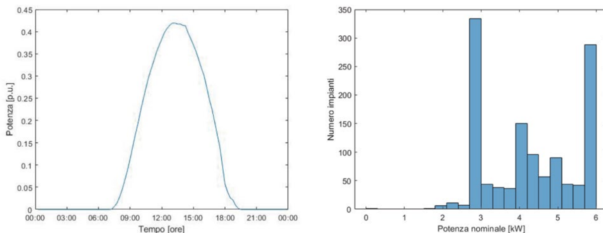
Figura 4.3 - Profilo di produzione in per unit degli impianti FV (figura a sinistra) e potenza nominale degli impianti considerati nell'aggregato (figura a destra)
