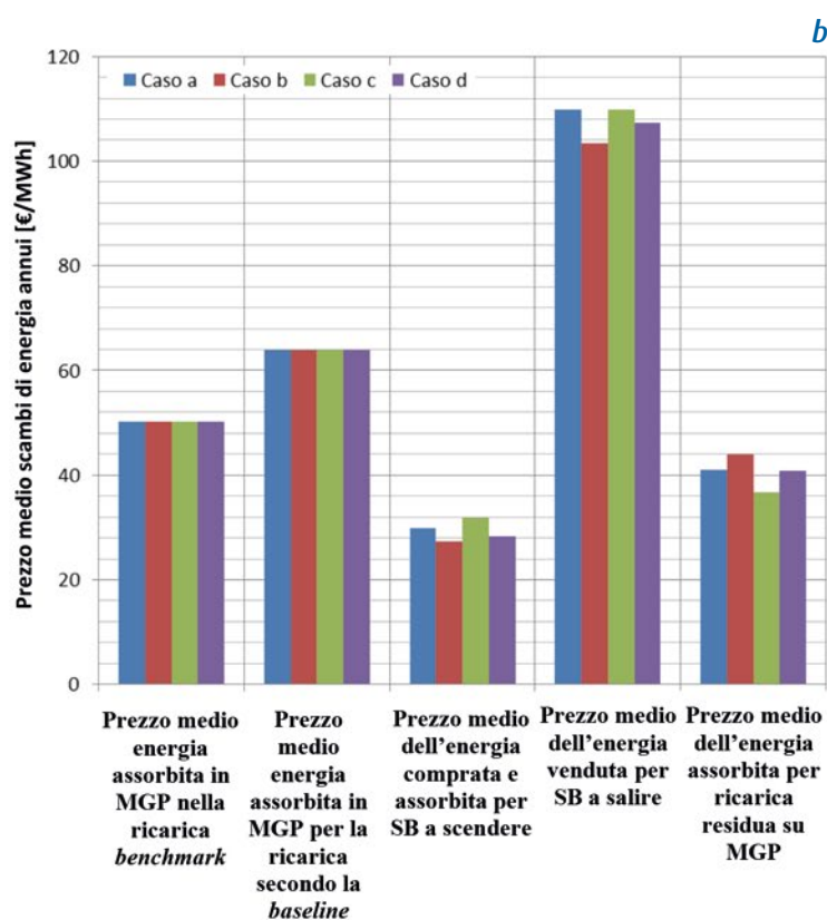
Figura 5.4 -Scambi di energia annui (a) e relativi prezzi medi unitari (b) per i casi di studio domestici e aziendali analizzati, con riferimento al periodo 1/8/2016 – 31/7/2017
