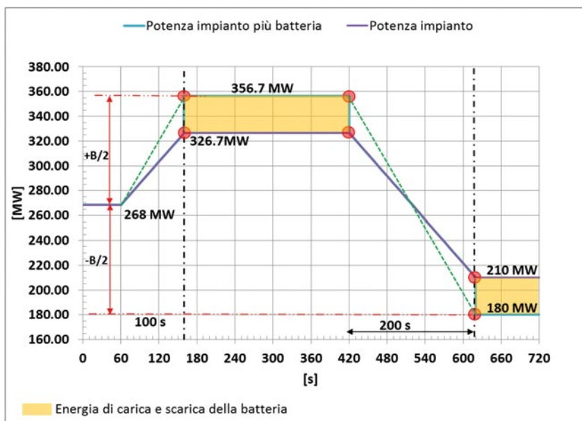
Figura 1.9 - Dinamica di erogazione dell'intera banda di regolazione di frequenza
