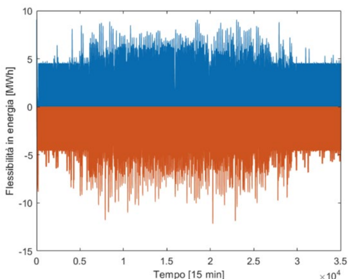
Figura 4.9 - Flessibilità in energia teorica dell'aggregato su un orizzonte temporale di un anno nel caso di funzionalità di autoconsumo con ricarica notturna
