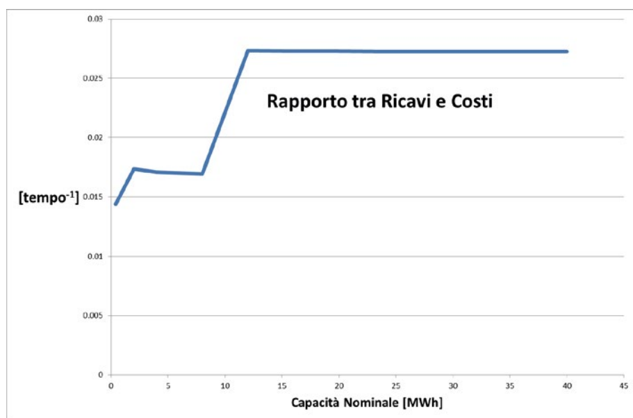
Figura 2.12 – Andamento del rapporto ricavi netti/costi di investimento al variare della taglia del SdA – caso di installazione nella zona SUD
