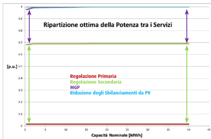
Figura 2.3 - Ripartizione ottima della potenza installata fra i vari servizi al variare della taglia - zona NORD con accoppiamento ad un impianto FV
