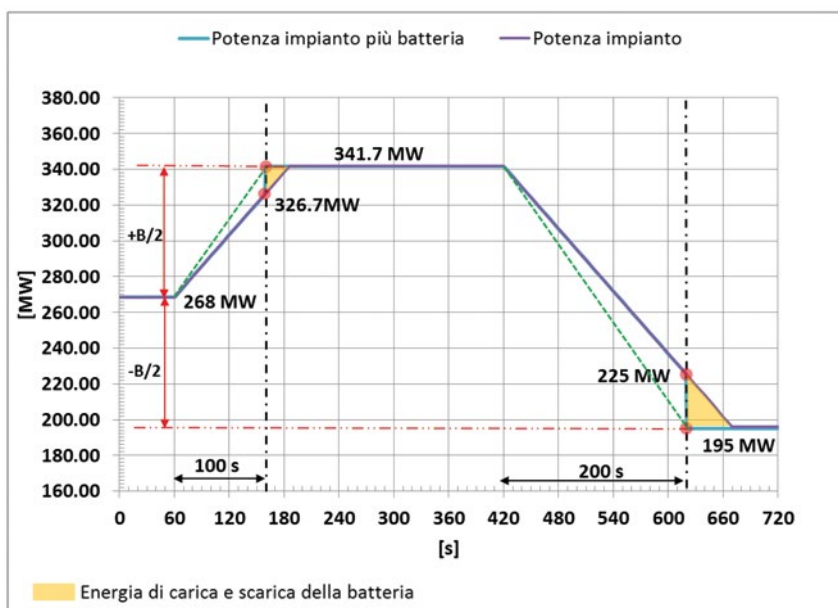
Figura 1.10 - Incremento della banda di regolazione secondaria con utilizzo della batteria in prossimità della fine rampa
