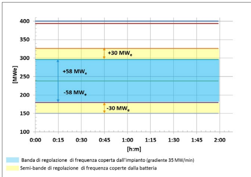
Figura 1.8 - Banda totale di regolazione di frequenza data dalla batteria e dal contributo massimo dell'impianto
