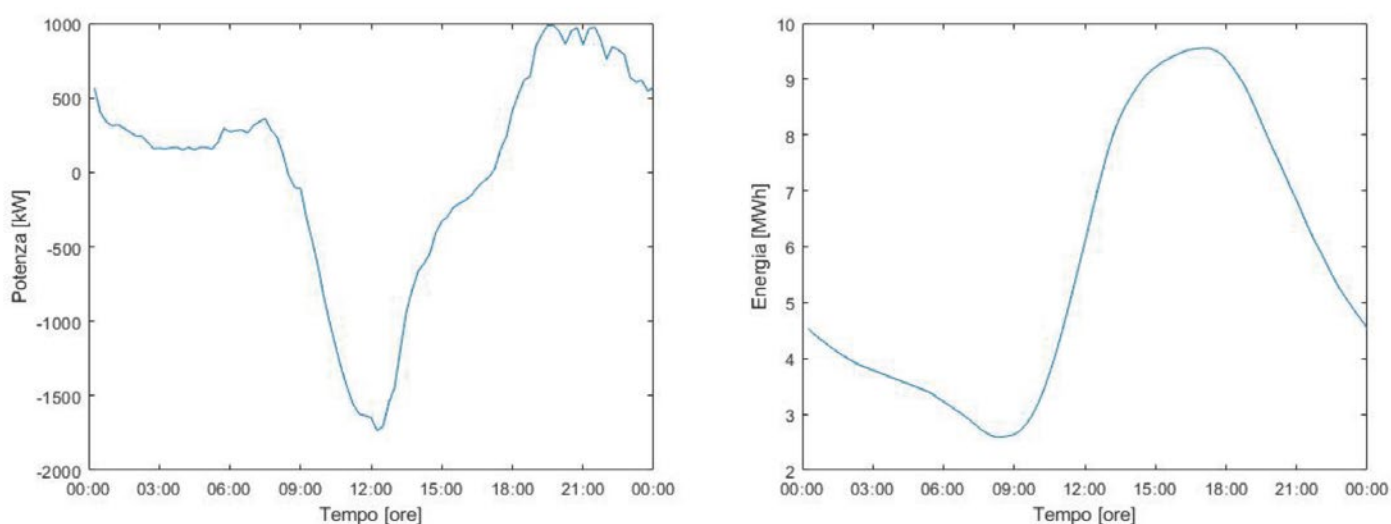
Figura 4.6 - Profilo della baseline in potenza ed energia dell'aggregato
