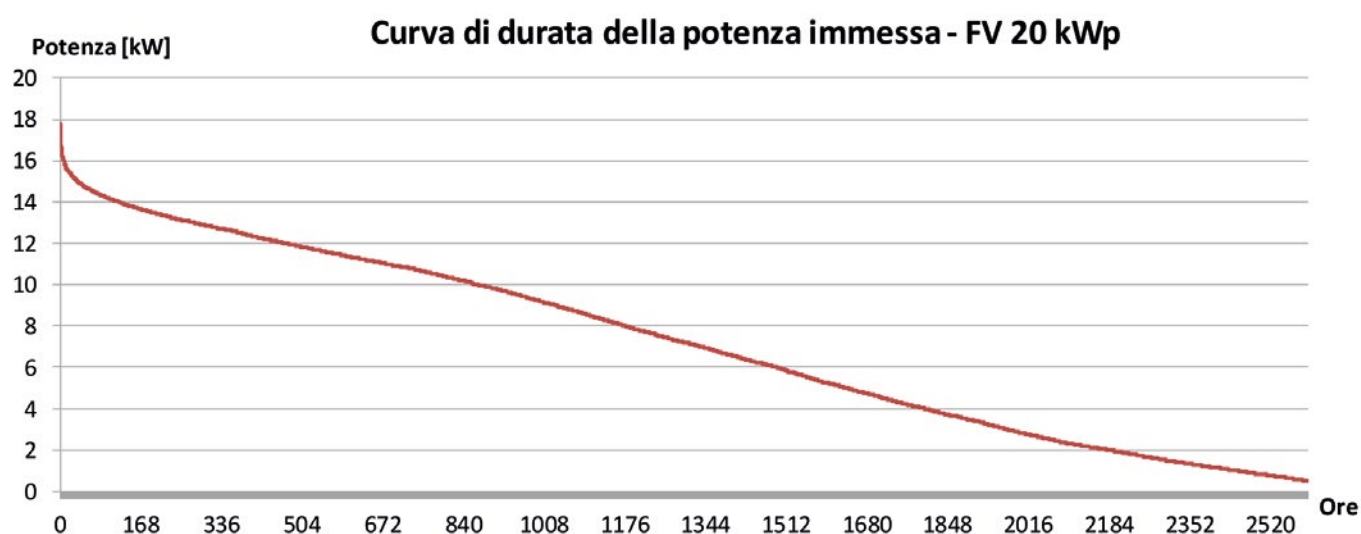
Figura 3.4 – Curva di durata della potenza immessa in rete dall'impianto di generazione.
