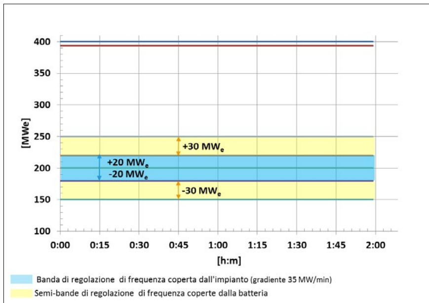
Figura 1.7 - Banda totale di regolazione di frequenza ottenuta come somma del contributo massimo della batteria e di un contributo parziale dell'impianto
