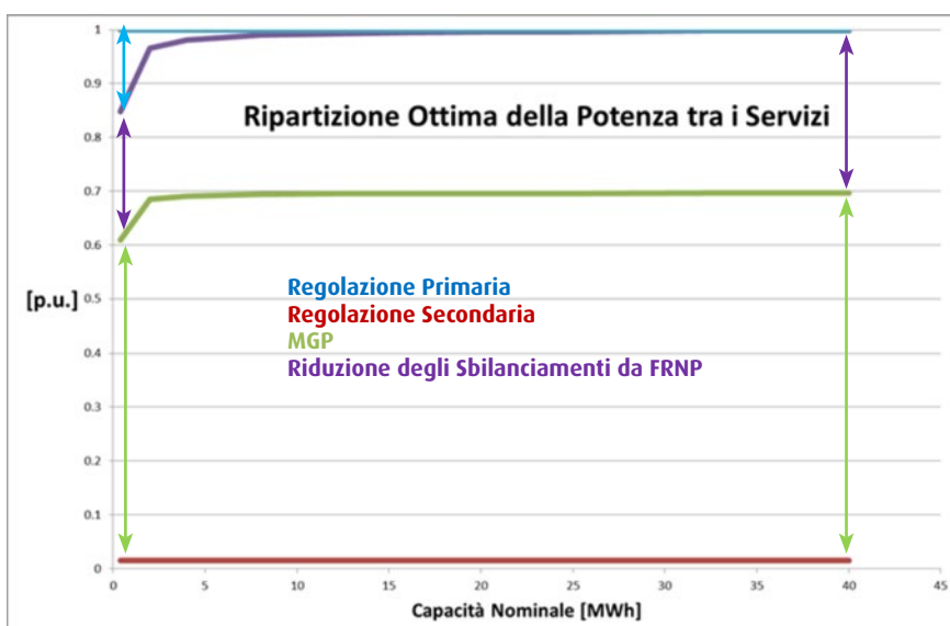
Figura 2.7 – Ripartizione della Potenza installata fra i vari servizi al variare della taglia – caso di installazione nella zona CNOR
