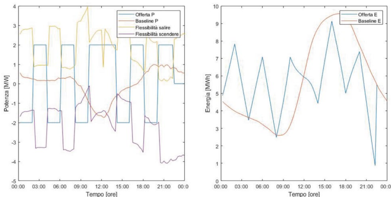
Figura 4.10 - Andamento della potenza ed energia dell'aggregato a fronte di un servizio di bilanciamento durante un giorno soleggiato estivo
