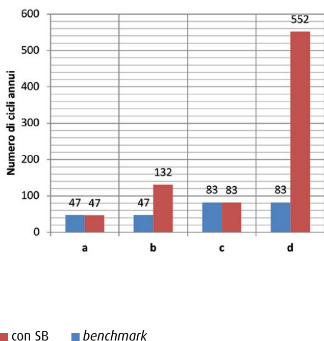
Figura 5.5 - Numero annuale di cicli equivalenti di carica-scarica a cui è sottoposta la batteria del VE: confronto tra valori benchmark (ossia senza svolgimento del SB) e valori in caso di svolgimento del SB
