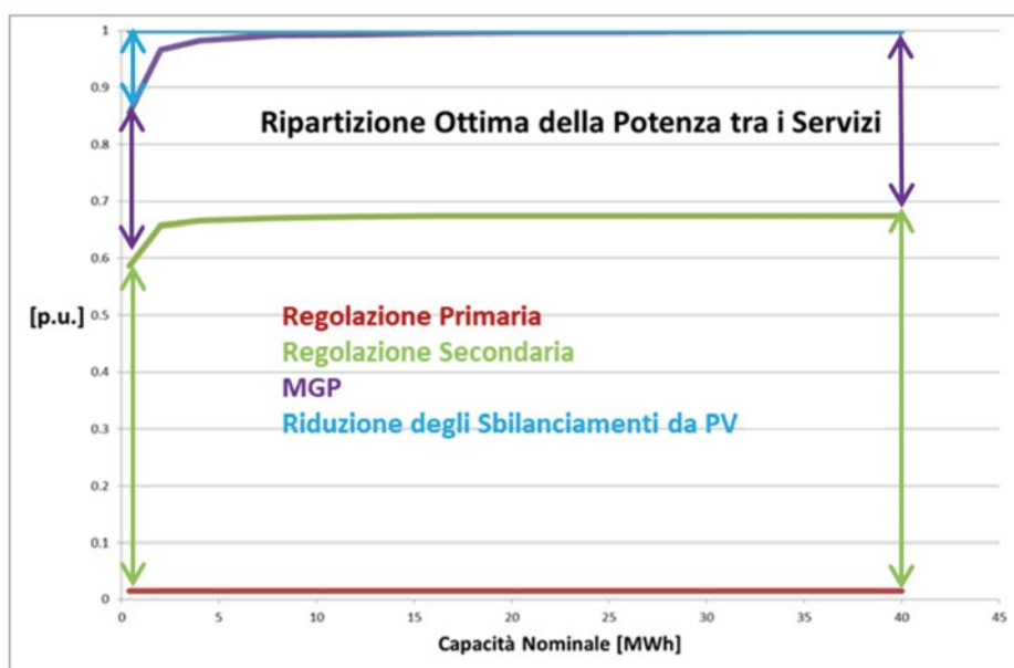
Figura 2.13 – Ripartizione della Potenza installata fra i vari servizi al variare della taglia – caso di installazione nella zona SUD
