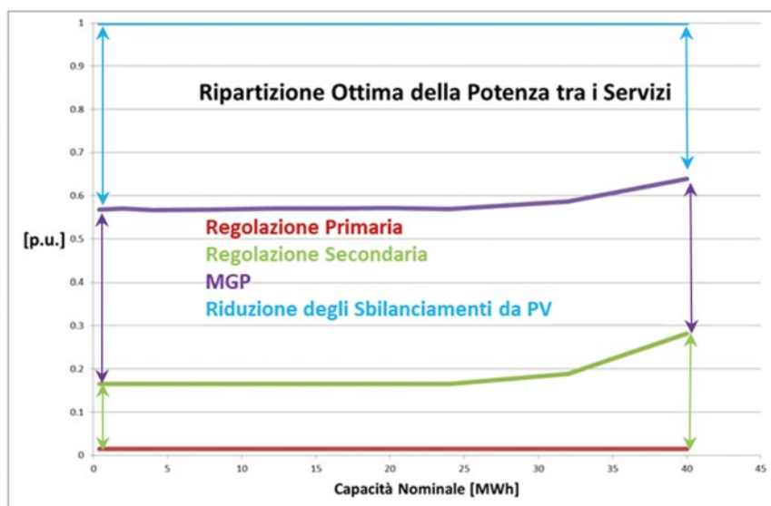
Figura 2.15 – Ripartizione ottima della potenza installata fra i vari servizi al variare della taglia – zona SUD con accoppiamento ad un impianto eolico
