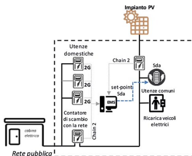
Figura 3.3 – Gestione ottimizzata di un SdA e della ricarica del veicolo elettrico per l'incremento dell'autoconsumo condominiale.
