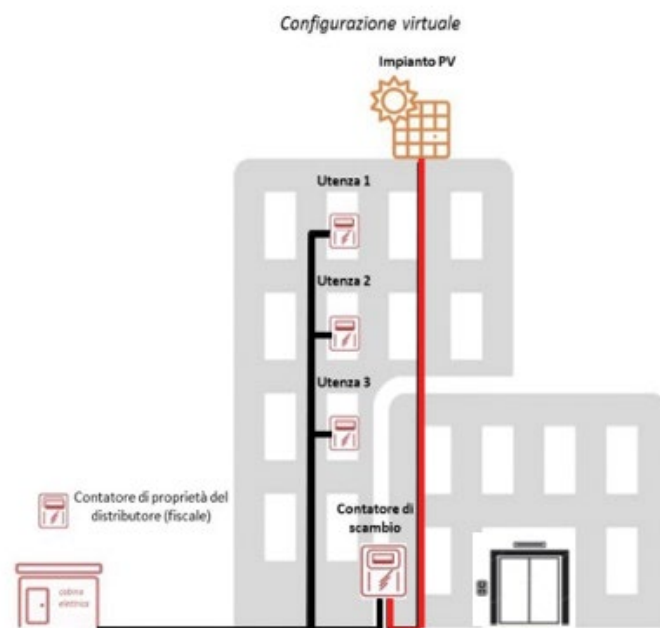
Figura 3.2 – Schema di autoconsumo “virtuale” con connessione tra utenze ed impianto di produzione mediante rete pubblica.
