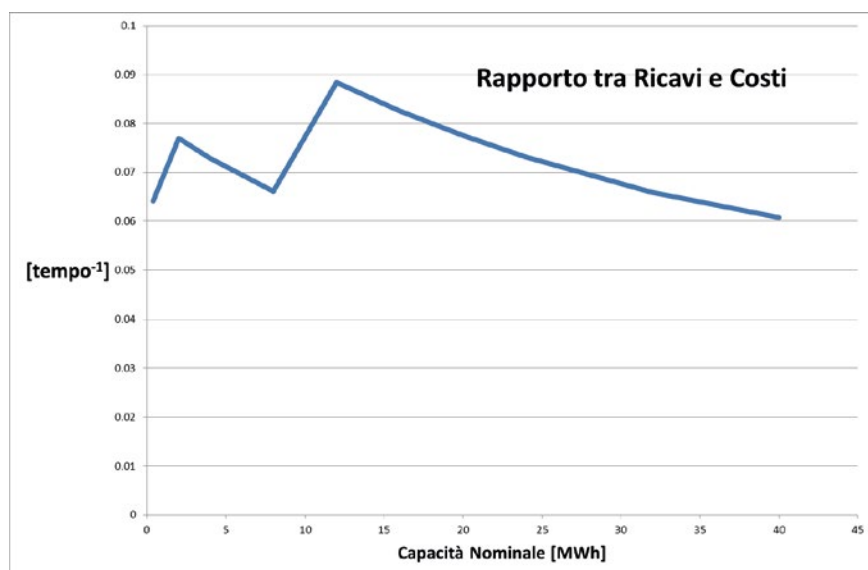
Figura 2.14 - Andamento del rapporto ricavi netti/costi di investimento al variare della taglia del SdA - zona SUD e accoppiamento con impianto eolico
