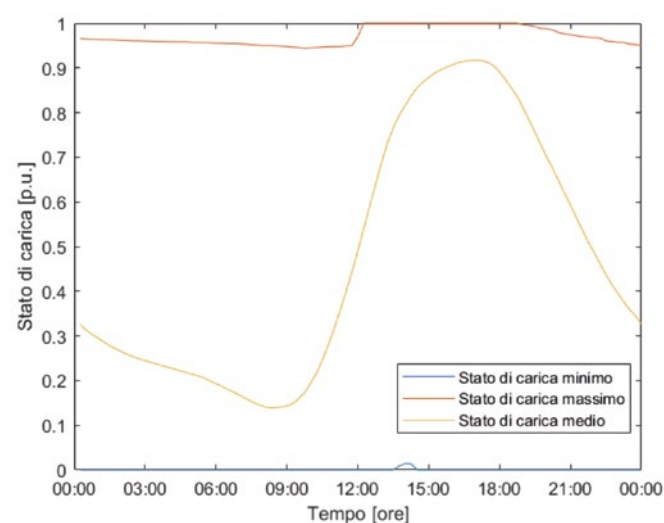
Figura 4.5 - Energia in per unit minima (linea blu), massima (linea rossa) e media (linea gialla) dei SdA nell'aggregato durante una giornata soleggiata feriale estiva
