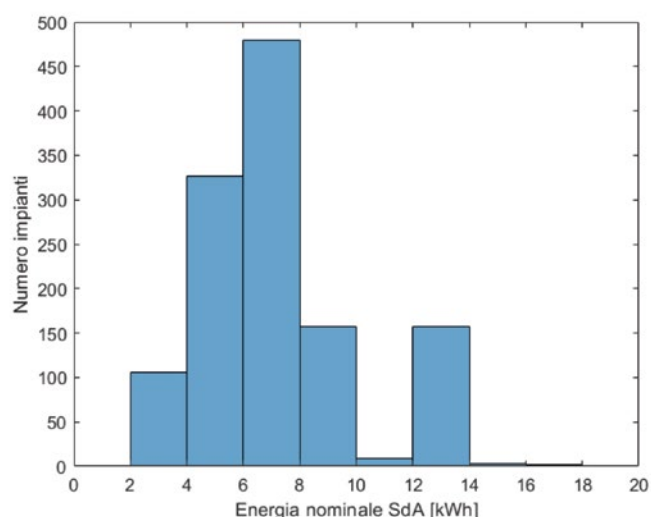
Figura 4.4 - Energia nominale dei SdA installati presso ogni utente nell'aggregato
